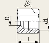
Union nuts to DIN 3870/ISO 8434-1
