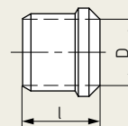
Cutting sleeves to DIN 3861/ISO 8434-1
